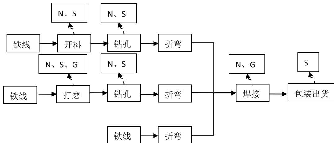
图 5-1 本项目生产工艺流程图
