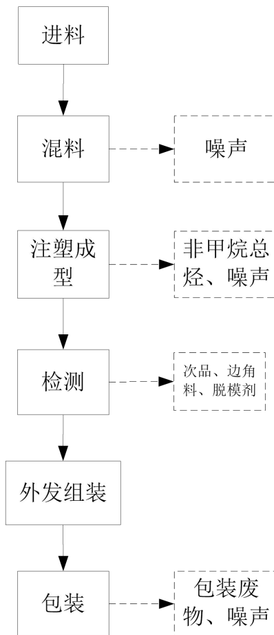
图 6-1 项目工艺流程图
