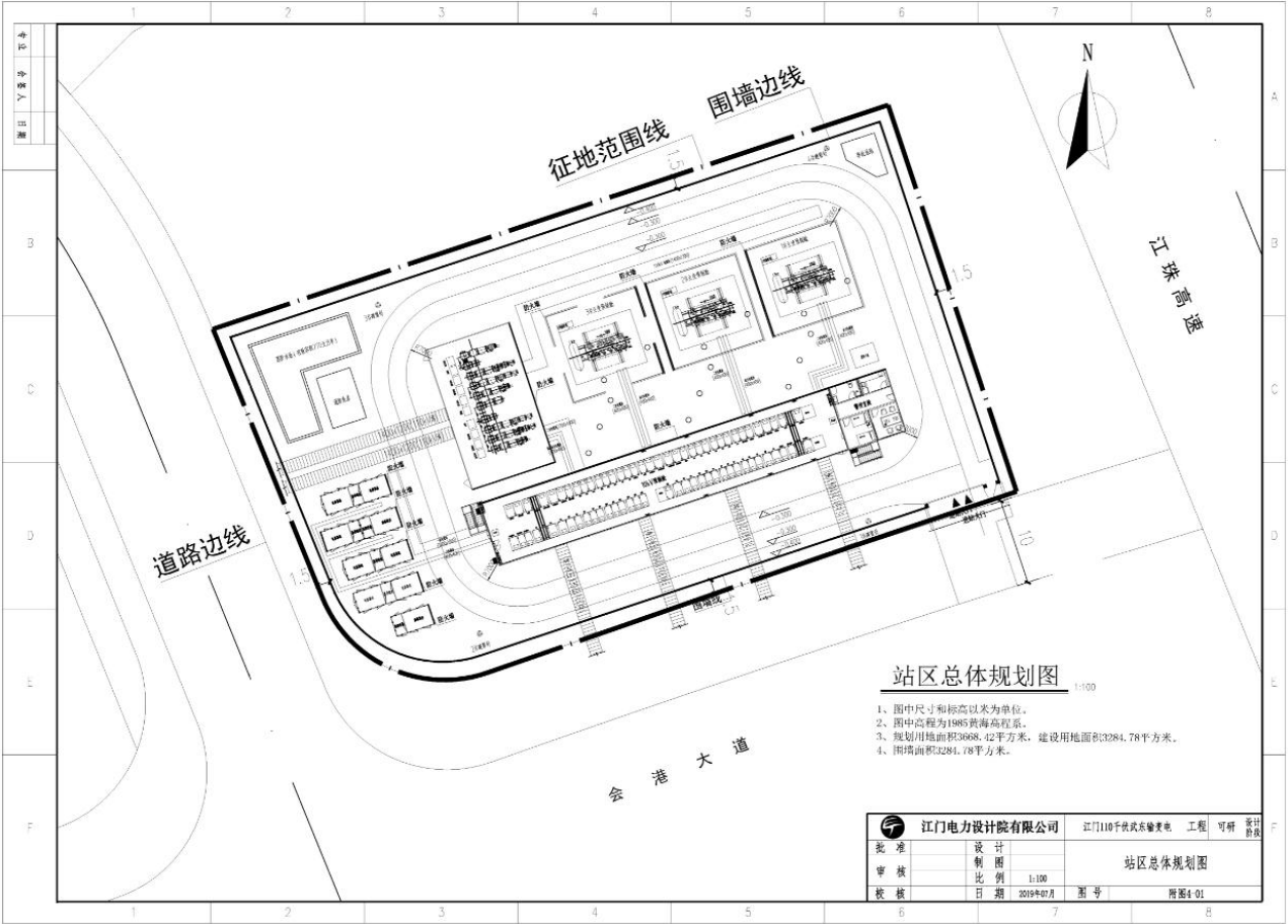
附图 3 站区总体规划图
