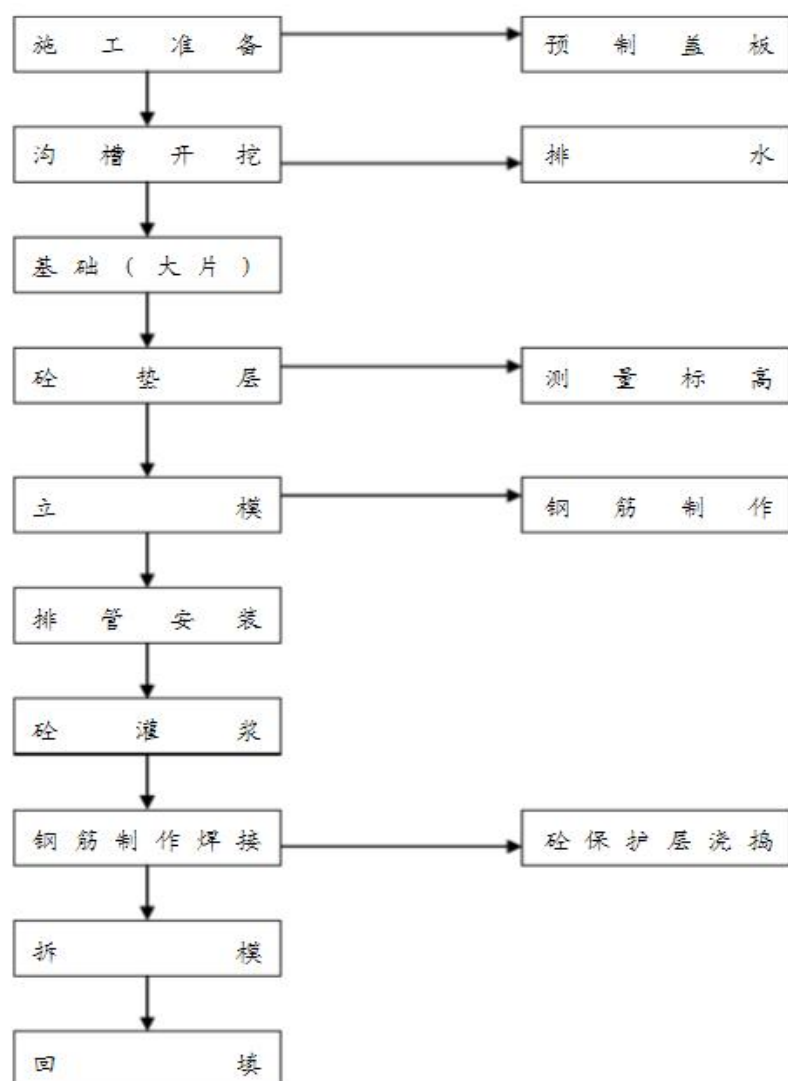
图 8.1-1 电缆沟施工工艺流程
