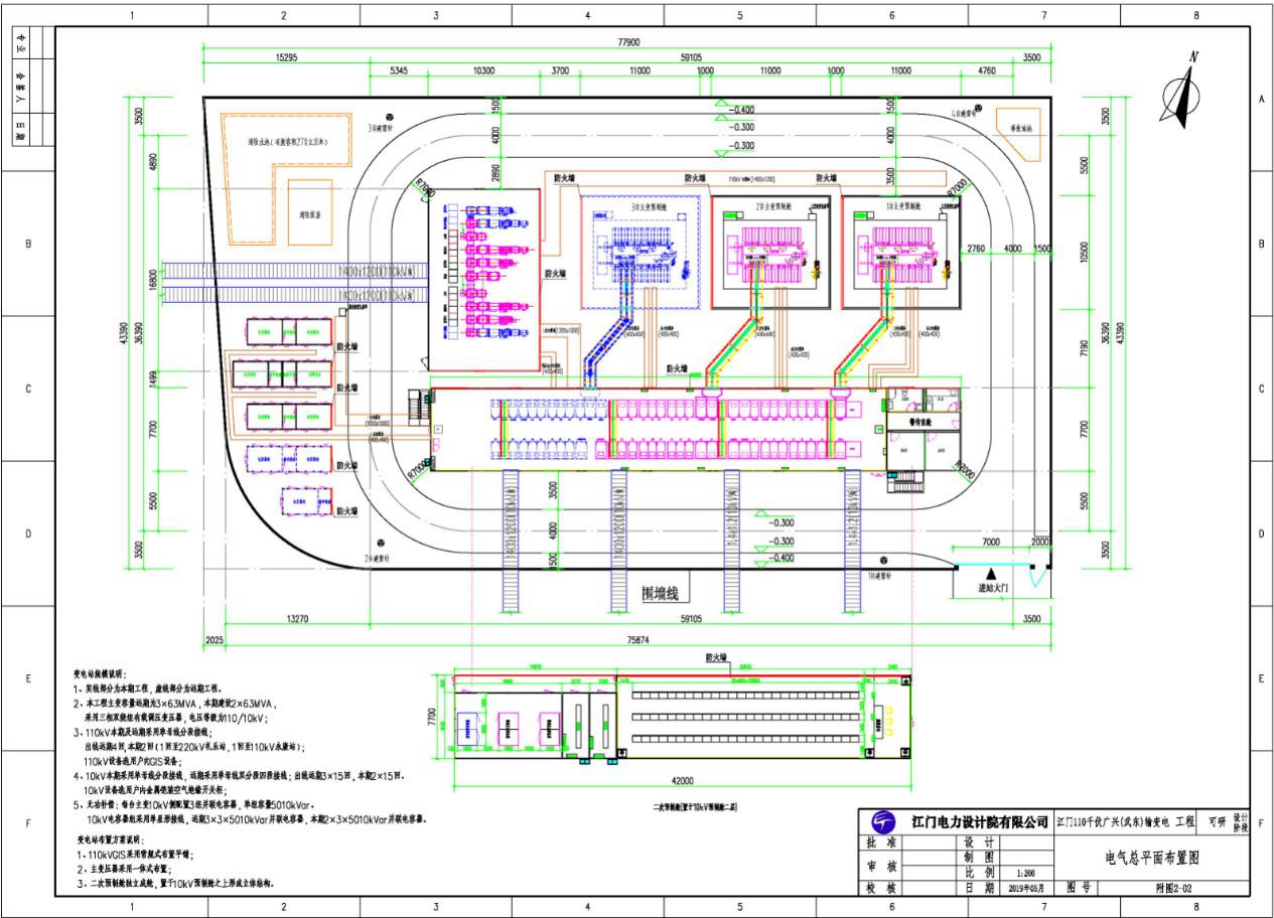
附图 1 变电站平面布置图
