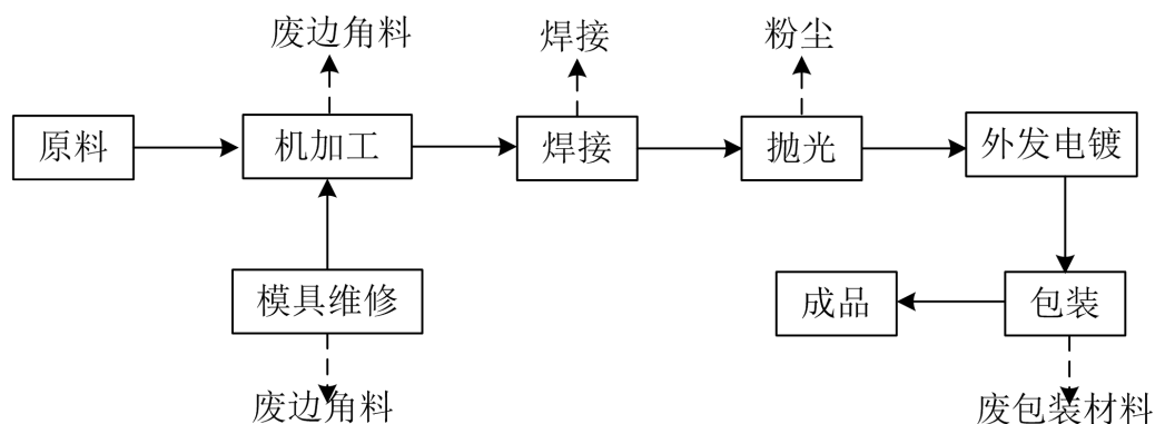
图 6-1 项目工艺流程图
