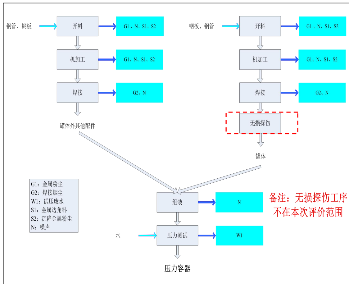
图-2 压力容器生产工艺流程及产污环节图
