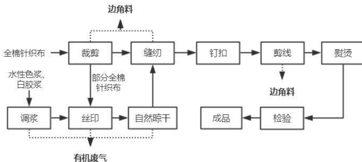
图 5-1 全棉针织婴儿连身衣、睡衣套装生产工艺流程图
