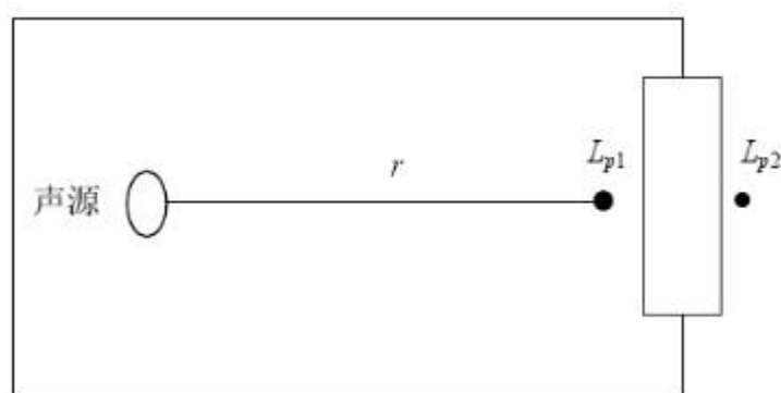
图 7-4 室内声源等效为室外声源图例
