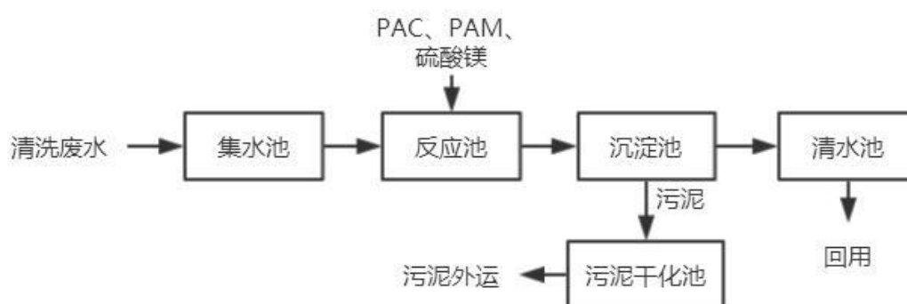
图 7-1 项目废水处理工艺流程图
