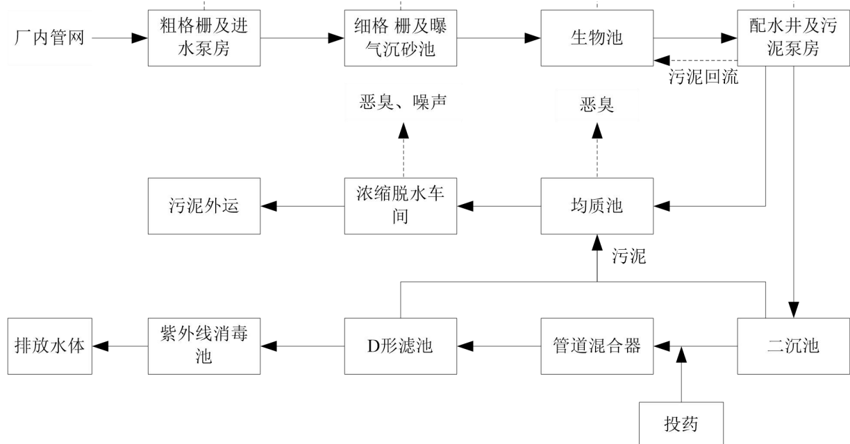
图 7-1 杜阮污水厂工艺流程图
