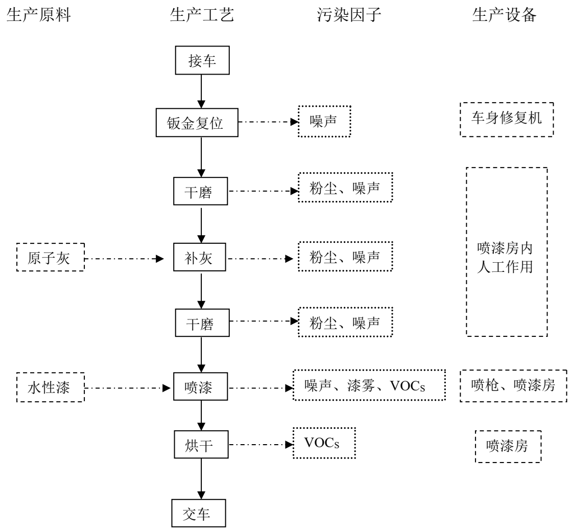
图 5-1 生产工艺流程图（本项目不设洗车工序）
