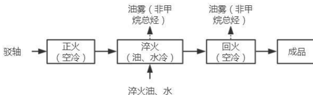
图 5-1 驳轴生产工艺流程图
