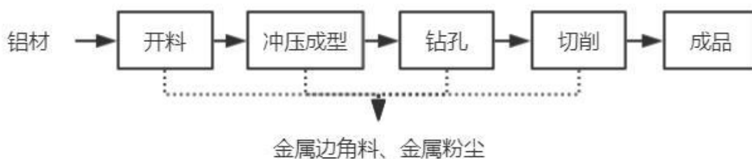
图 5-3 油缸生产工艺流程图
