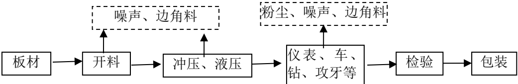
图 5-1 项目生产工艺流程及产污节点图
