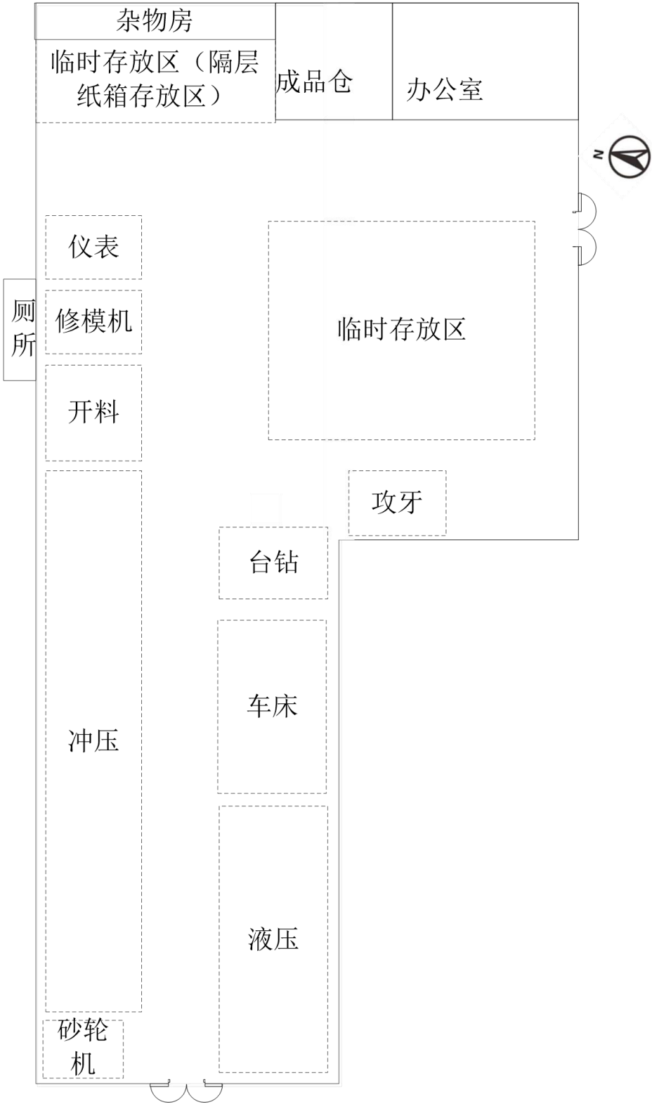
附图:4： 厂房平面布置图
