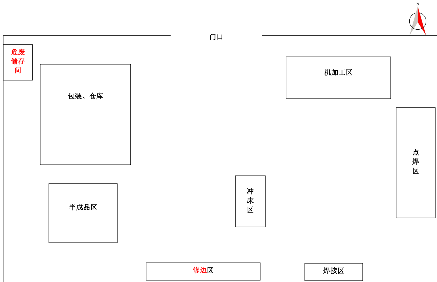
附图 4 项目厂区平面图
