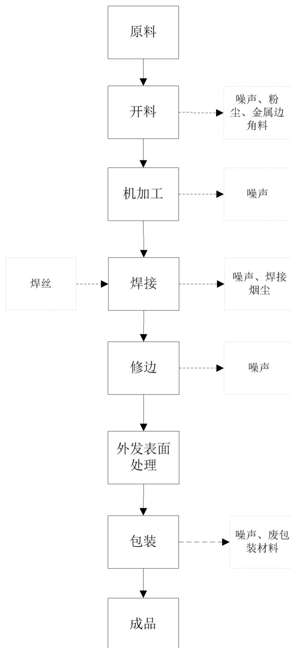
图 6-1 项目工艺流程图
