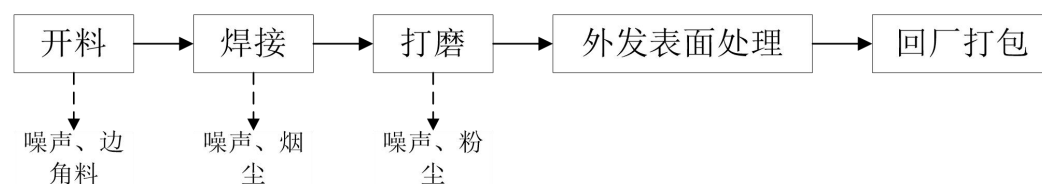
图1-1 项目生产工艺流程图
