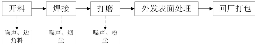
图 5-1 项目生产工艺流程图
