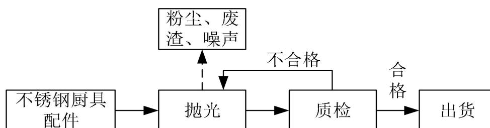
图 5-1 项目生产工艺流程及产污环节示意图
