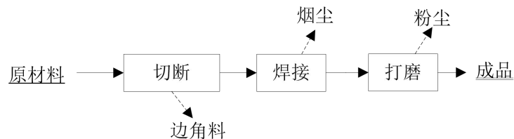
图6-2 臂杆生产工艺流程图
