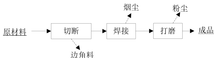
图2-2 臂杆生产工艺流程图
