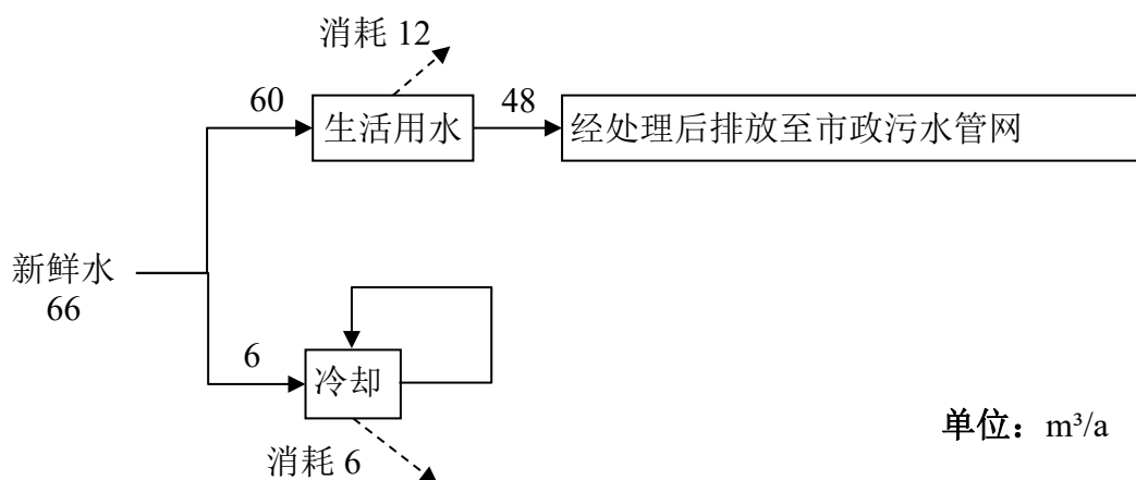
图1-1 水平衡图
