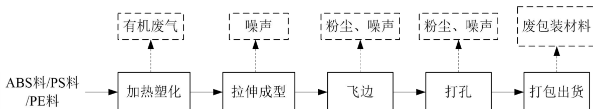
图1-2 项目生产工艺流程图
