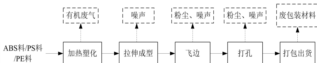
图 5-1 项目生产工艺流程图
