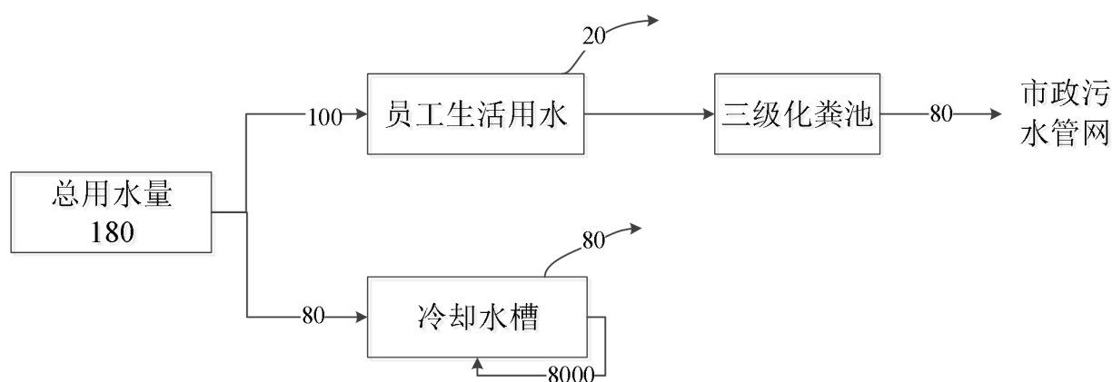
图 1-1 水平衡图 (m 3 /a)
