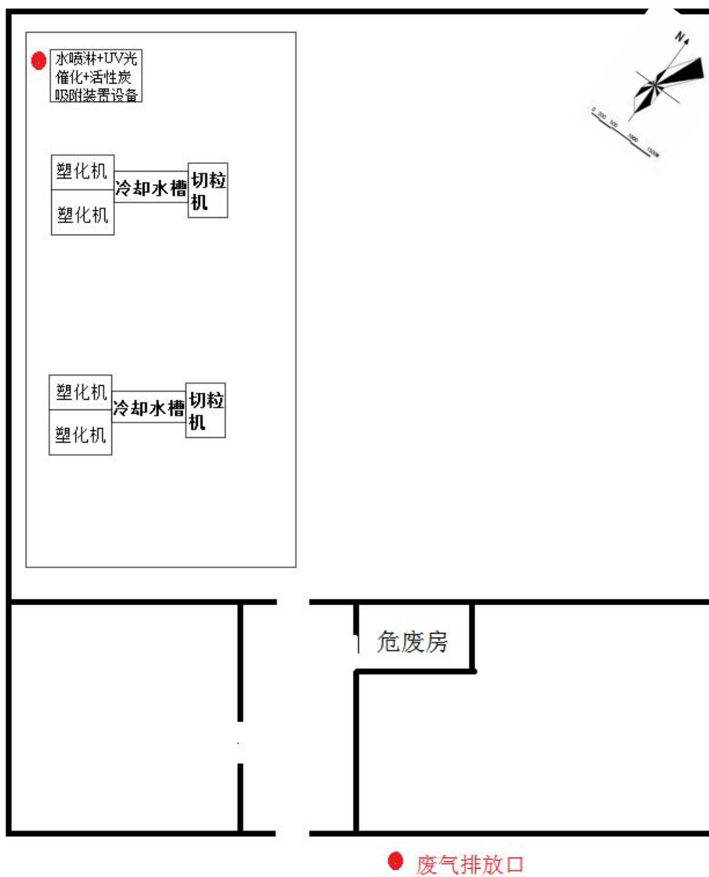
附图 4 总平面布置图
