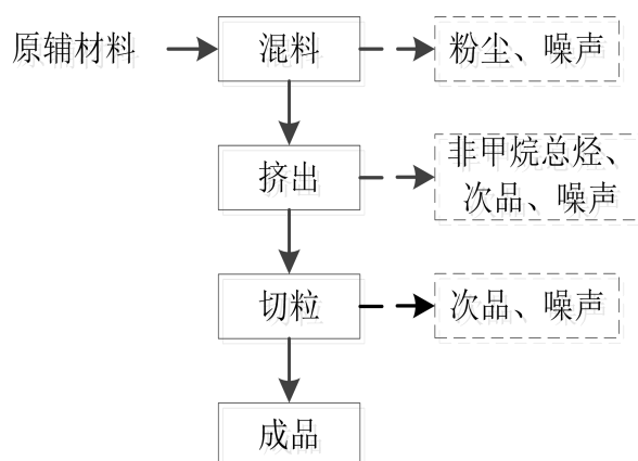
图 5-1 塑料生产工艺流程图
