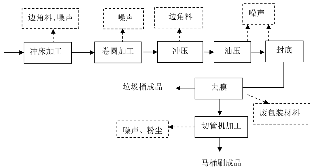
图 1 垃圾桶、马桶刷生产工艺流程图
