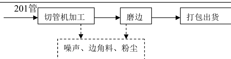
图3 马桶刷杯加工生产工艺流程图
