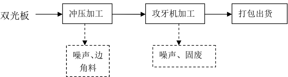
图2 镜配件加工生产工艺流程图
