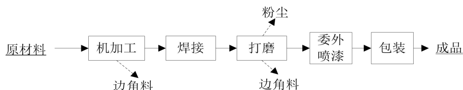
图2-1 项目生产工艺流程图
