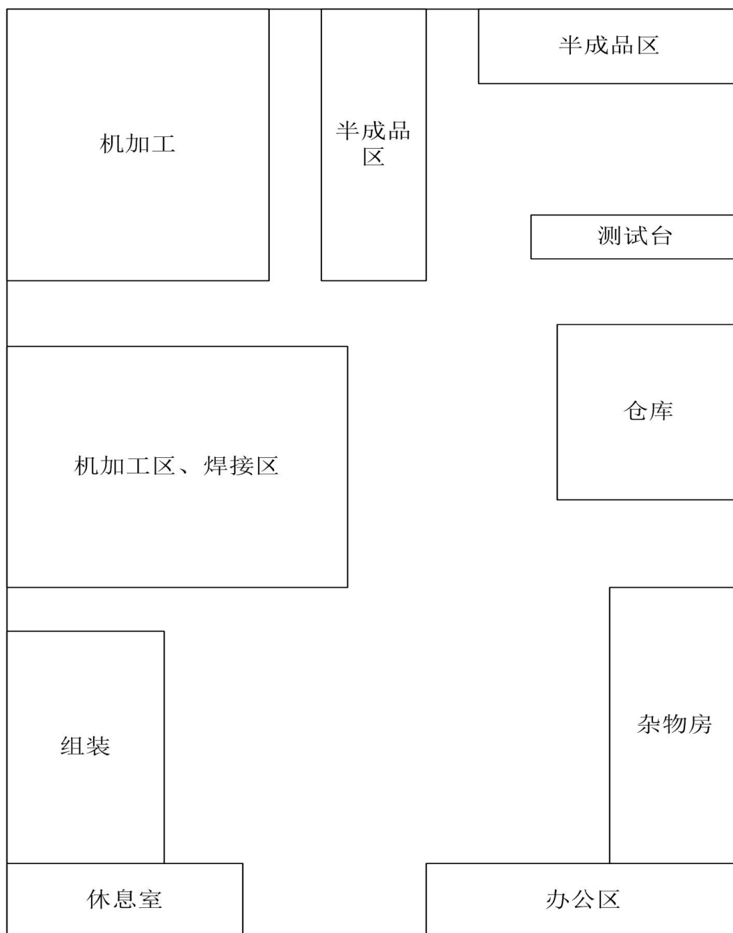
附图 4 项目厂区平面布置图
