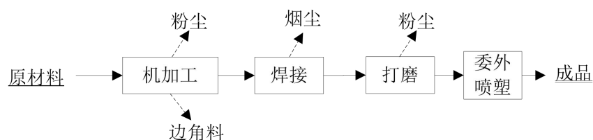
图6-1 项目生产工艺流程图
