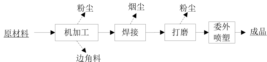
图2-1 项目生产工艺流程图
