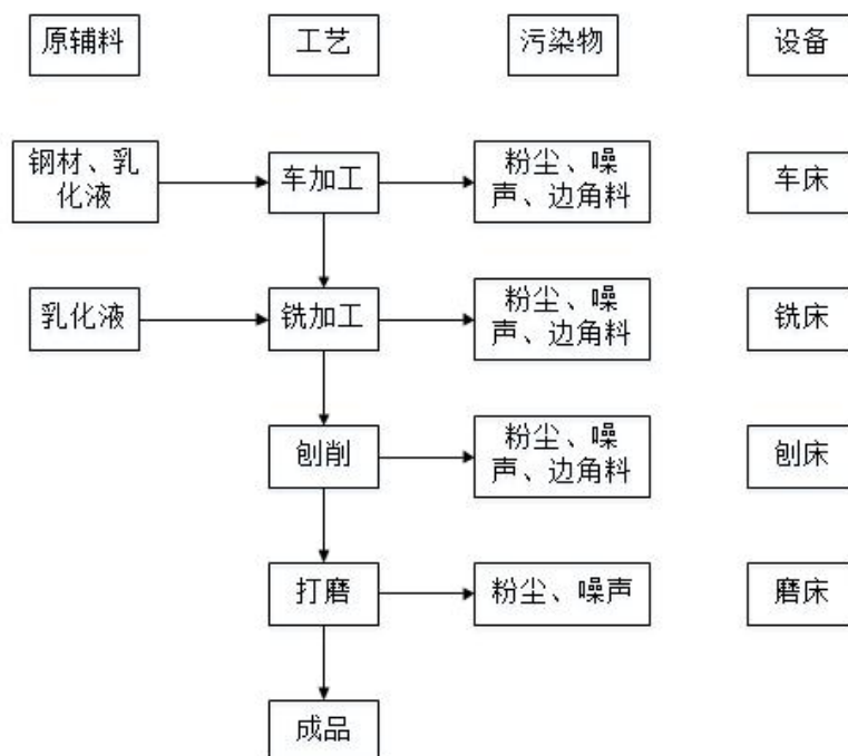
图 5-1 项目生产工艺流程及产污环节示意图
