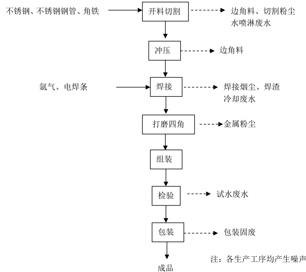
图 5-1 生产工艺流程图
