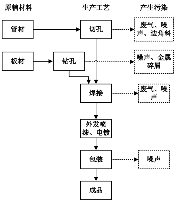
图 2-1 项目路灯生产工艺流程图
