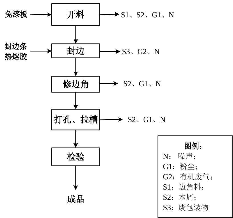
图-1 工艺流程图及产污环节图
