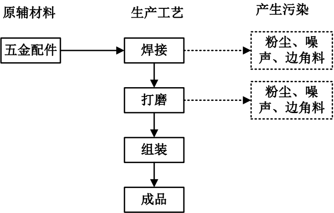
图 6-2 项目灯饰配件生产工艺流程图
