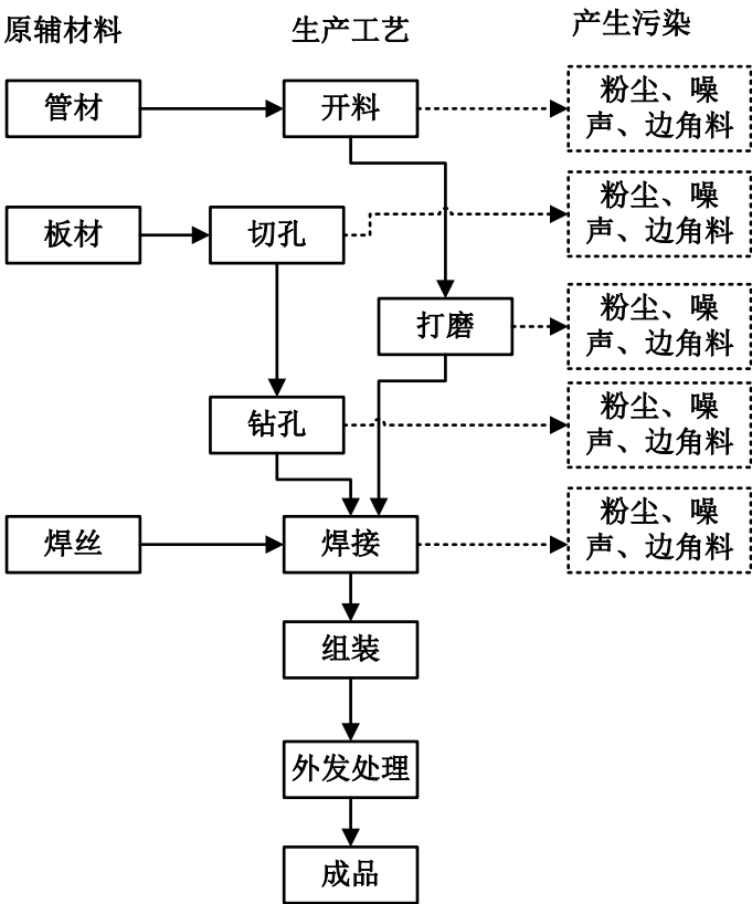
图 6-1 项目灯柱生产工艺流程图
