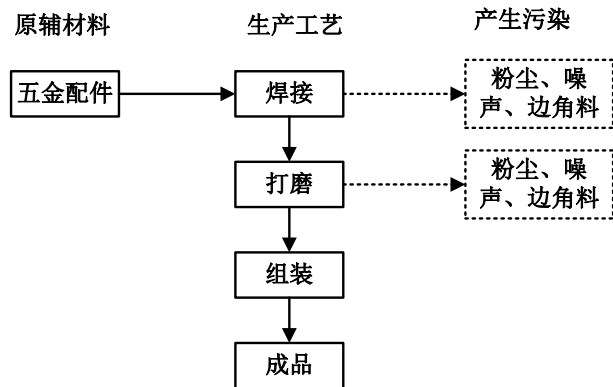
图 2-2 项目灯饰配件生产工艺流程图
