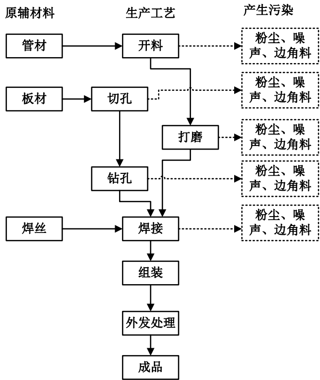
图 2-1 项目灯柱生产工艺流程图
