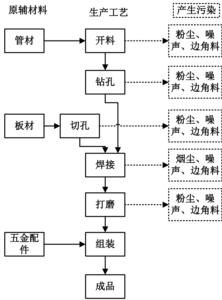
图 2-1 项目灯柱生产工艺流程图
