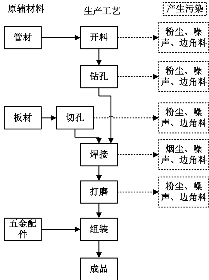
图 6-1 项目路灯生产工艺流程图
