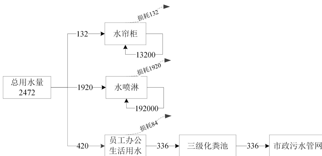
图 5-2 本项目水平衡图 (单位: m 3 /a)
