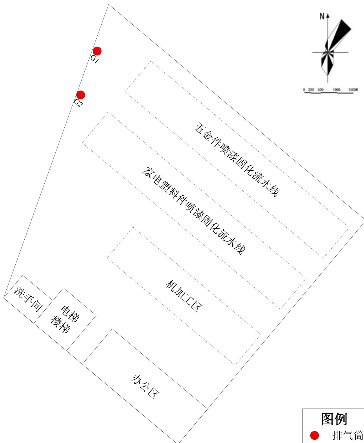
附图 4 项目厂区平面图
