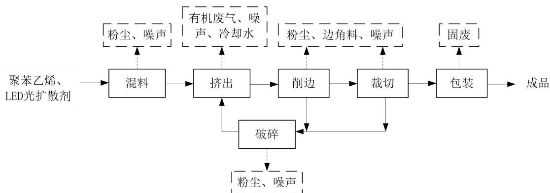
图1-2 项目生产工艺流程图
