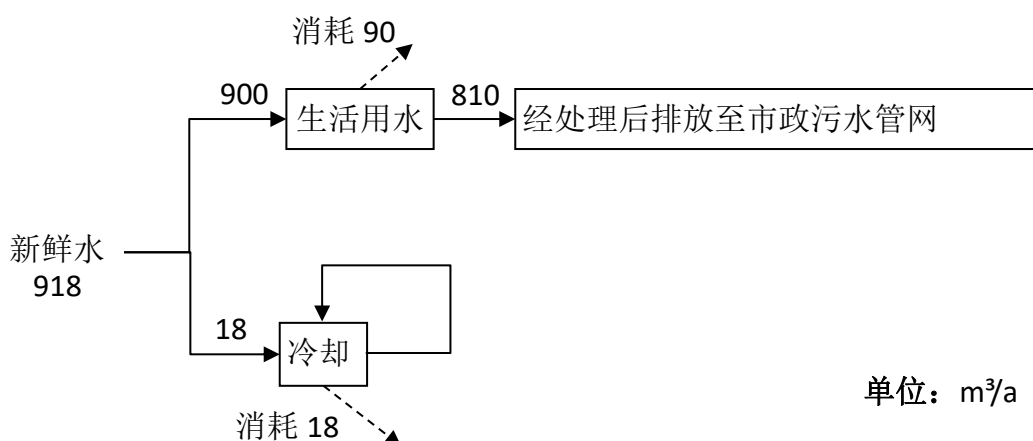
图1-1 水平衡图
