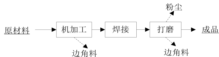
图2-1 项目生产工艺流程图
