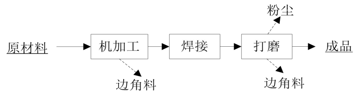
图6-1 项目生产工艺流程图
