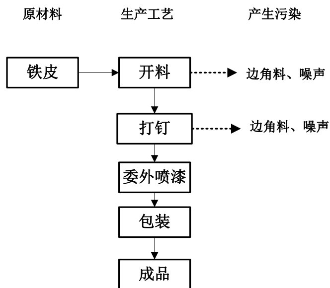
图6-1 生产工艺流程及产污环节示意图
