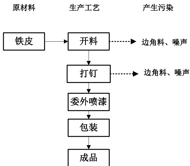
图2-1 生产工艺流程及产污环节示意图
