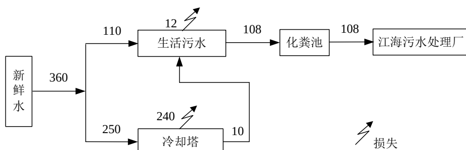
图 1-1 项目水平衡图 (t/a)
