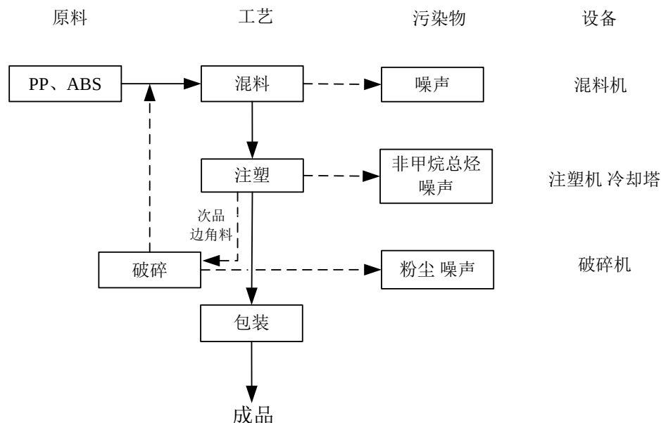
图 5-1 生产工艺流程图
