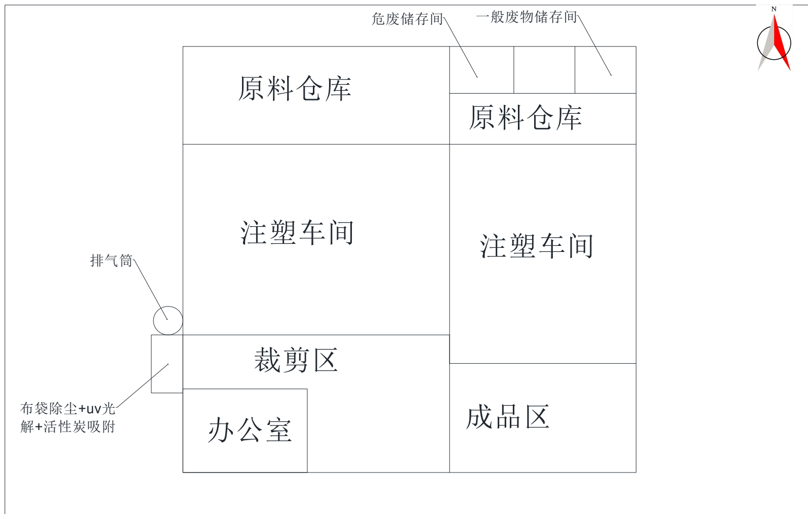
附图 4 项目厂区平面图
