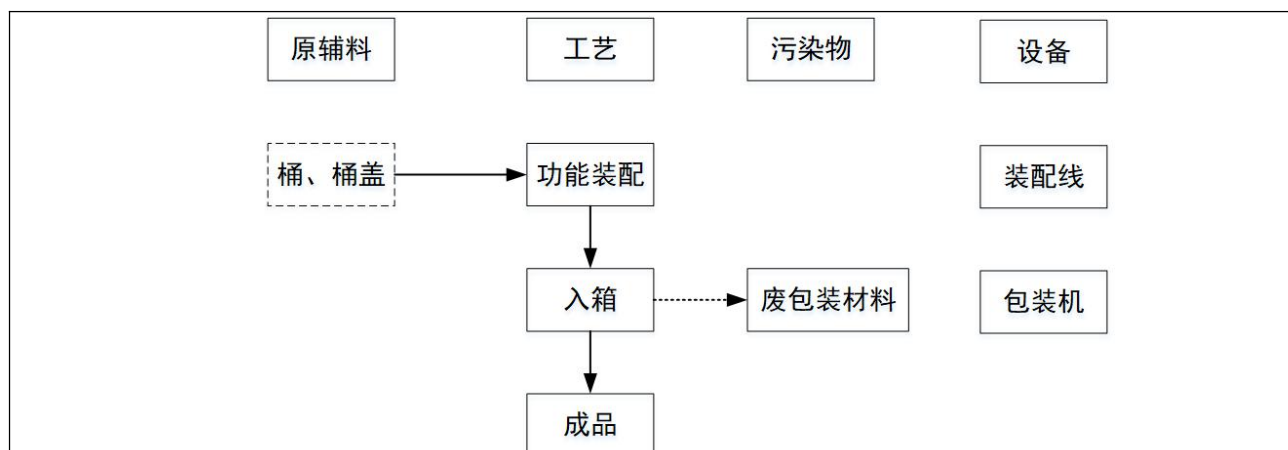
图 5-3 垃圾桶组装工艺流程及产污环节示意图
