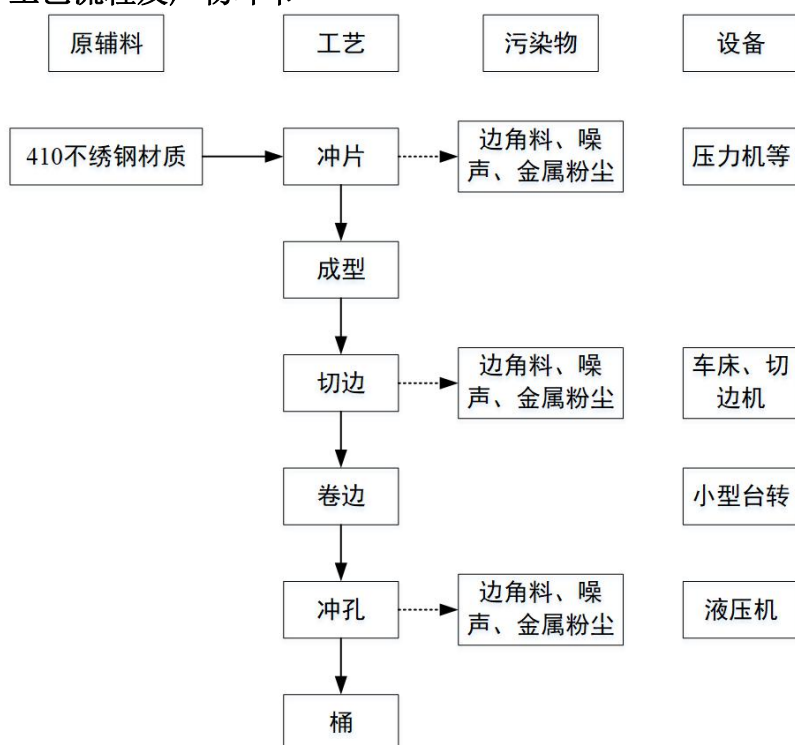
图 5-1 垃圾桶制造工艺流程及产污环节示意图
