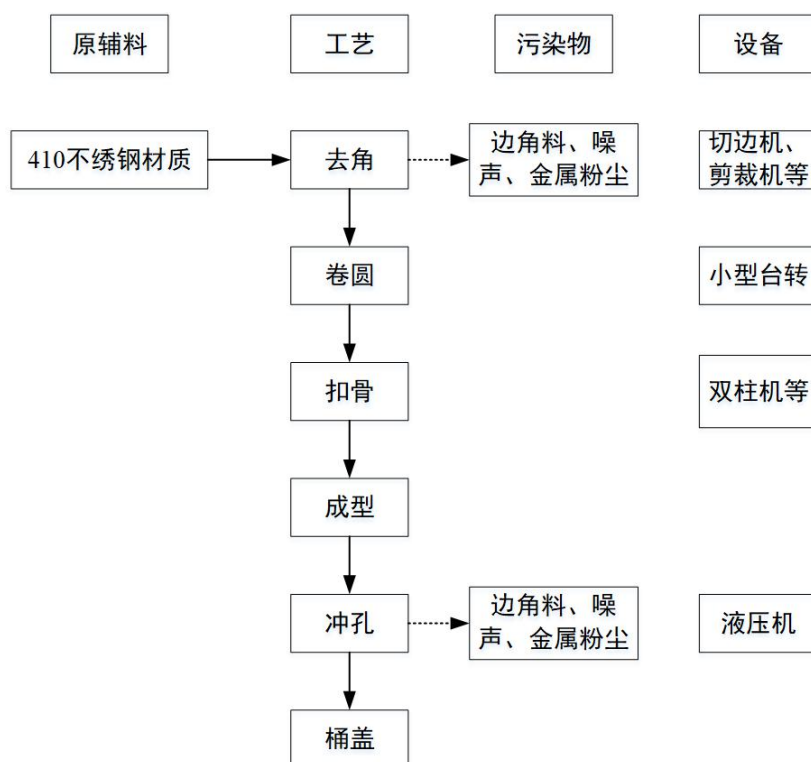
图 5-2 垃圾桶盖制造工艺流程及产污环节示意图
