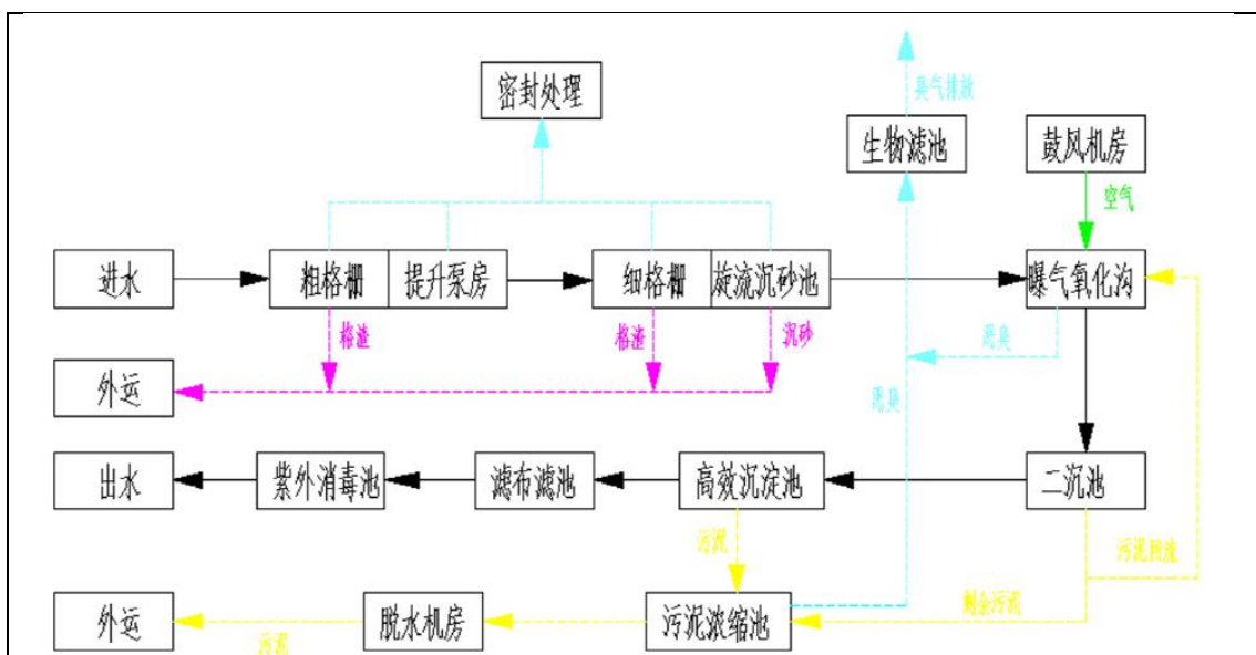
图 7-1 迳头污水处理厂提标改造后废水处理工艺
