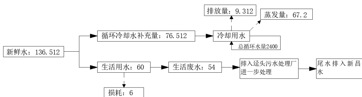
图 1-1 项目水平衡图（单位：m³/a）
