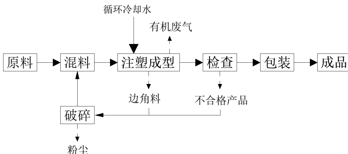
图5-2 塑料制品生产工艺及产污环节图
