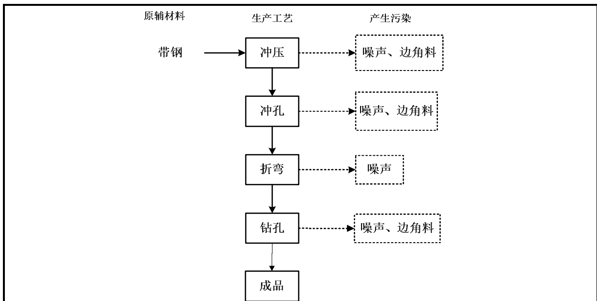
图 2-1 项目工艺流程图
