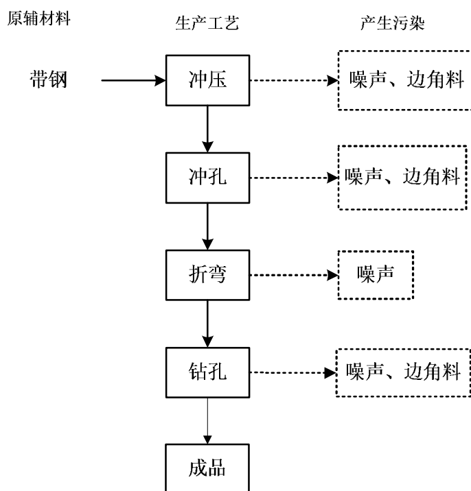
图 6-1 项目工艺流程图
