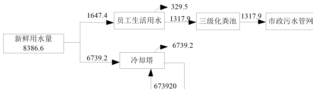
图 1-1 水平衡图 (m 3 /a)
