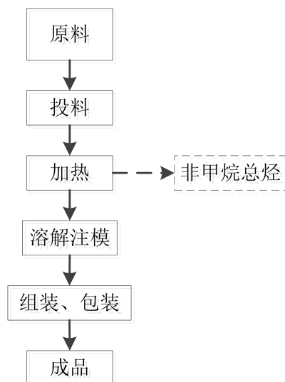
图 5-2 精密注塑件生产工艺流程图
