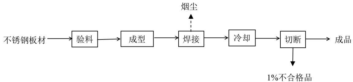
图 5-1 项目生产工艺流程图
