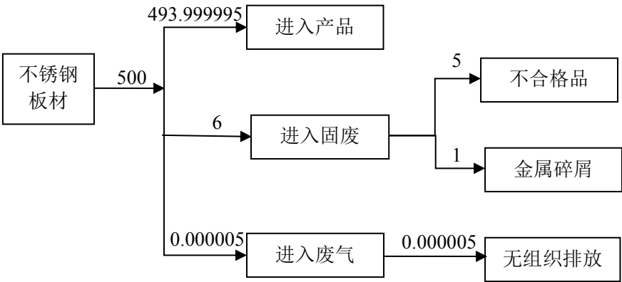
图 1-2 本项目物料平衡（t/a）
