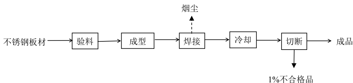
图 1-3 不锈钢管生产工艺流程图
