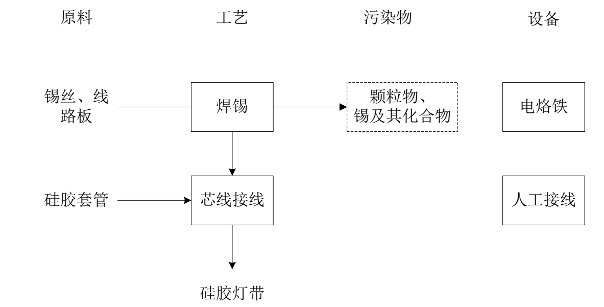
图 3 硅胶灯带生产工艺流程图
