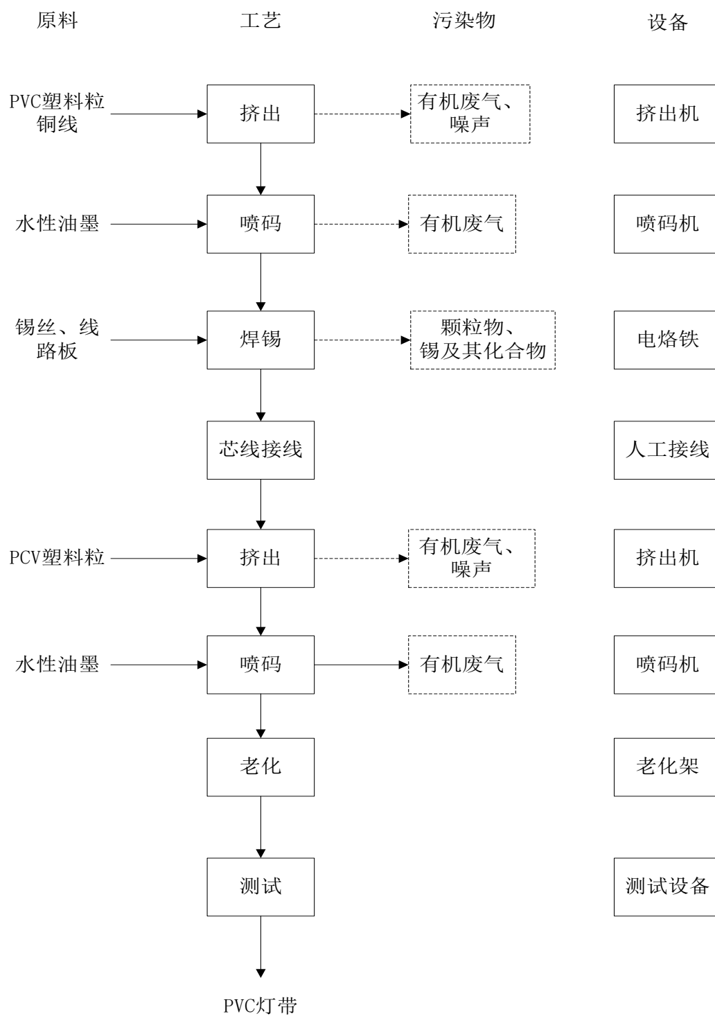
图2 PVC灯带生产工艺流程图
