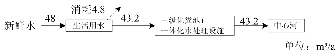
图1-1 整改后水平衡图
