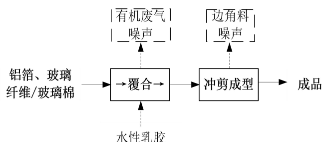
图1-2 保温棉生产工艺流程图
