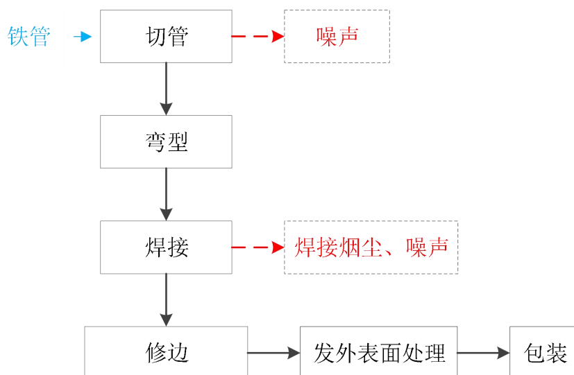
图 5-2 生产工艺流程图（2#）
