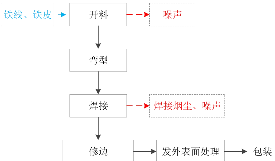
图 5-1 生产工艺流程图（1#）
