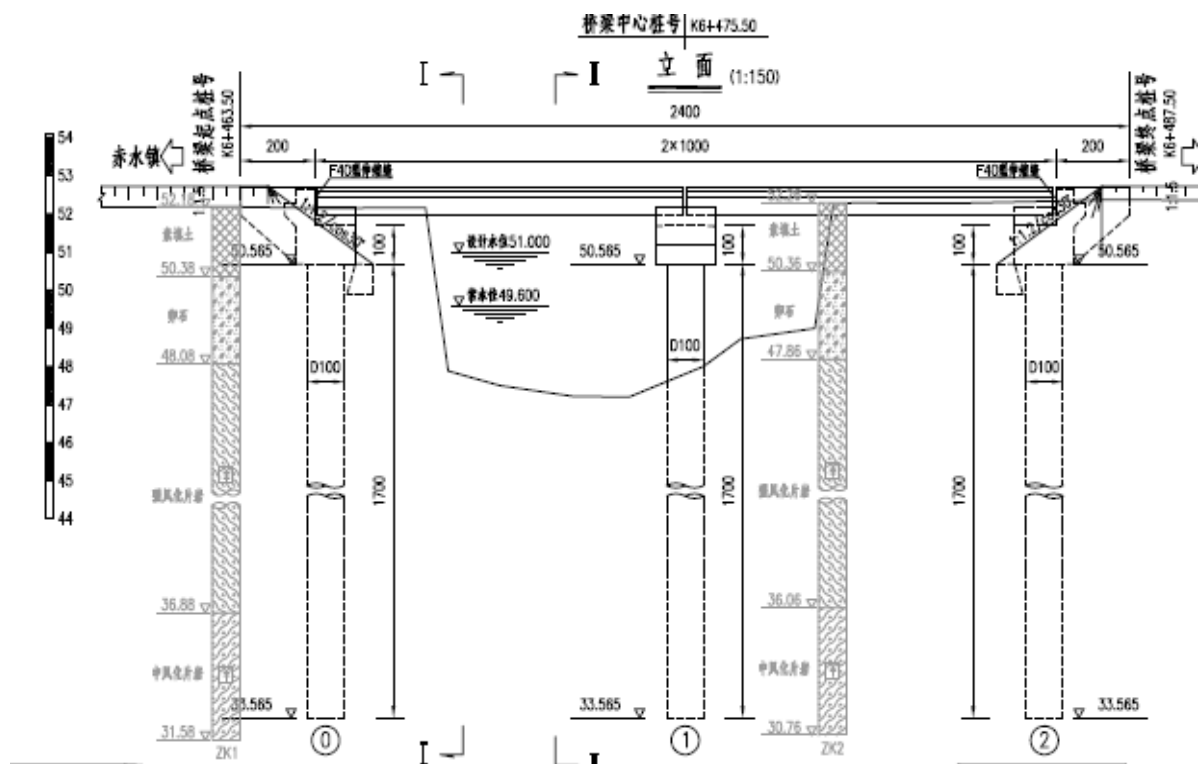
图 1-2 本项目桥梁立面设计图
