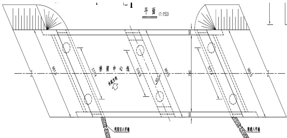
图 1-3 本项目桥梁平面设计图
