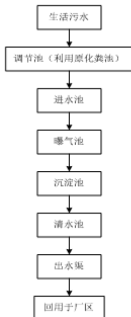
图 8-2 废水处理工艺流程图
