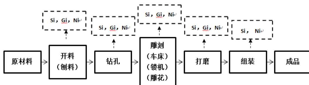
图 2-1 生产工艺流程
