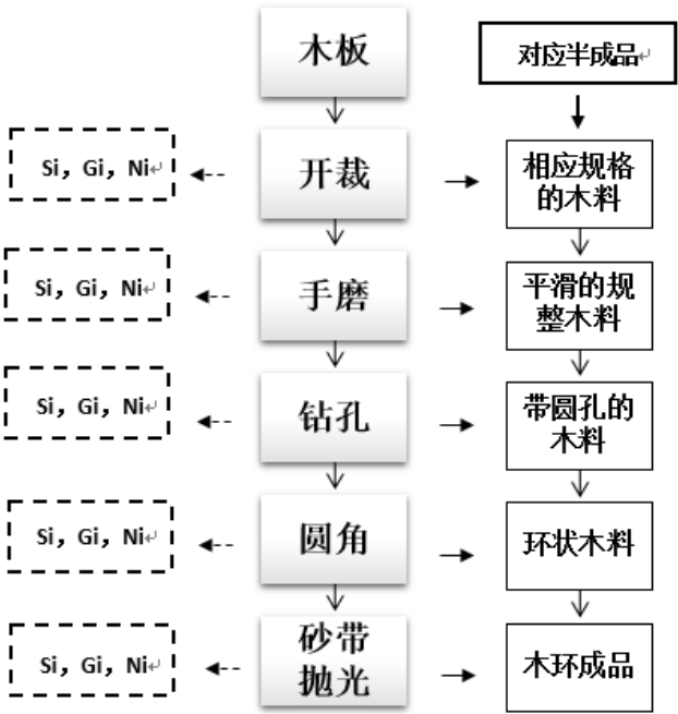
图 2-1 生产工艺流程
