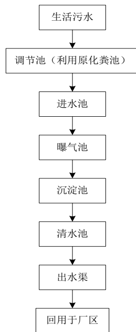
图 8-1 废水处理工艺流程图
