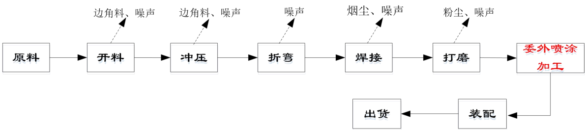
图 6-1 项目工艺流程图
