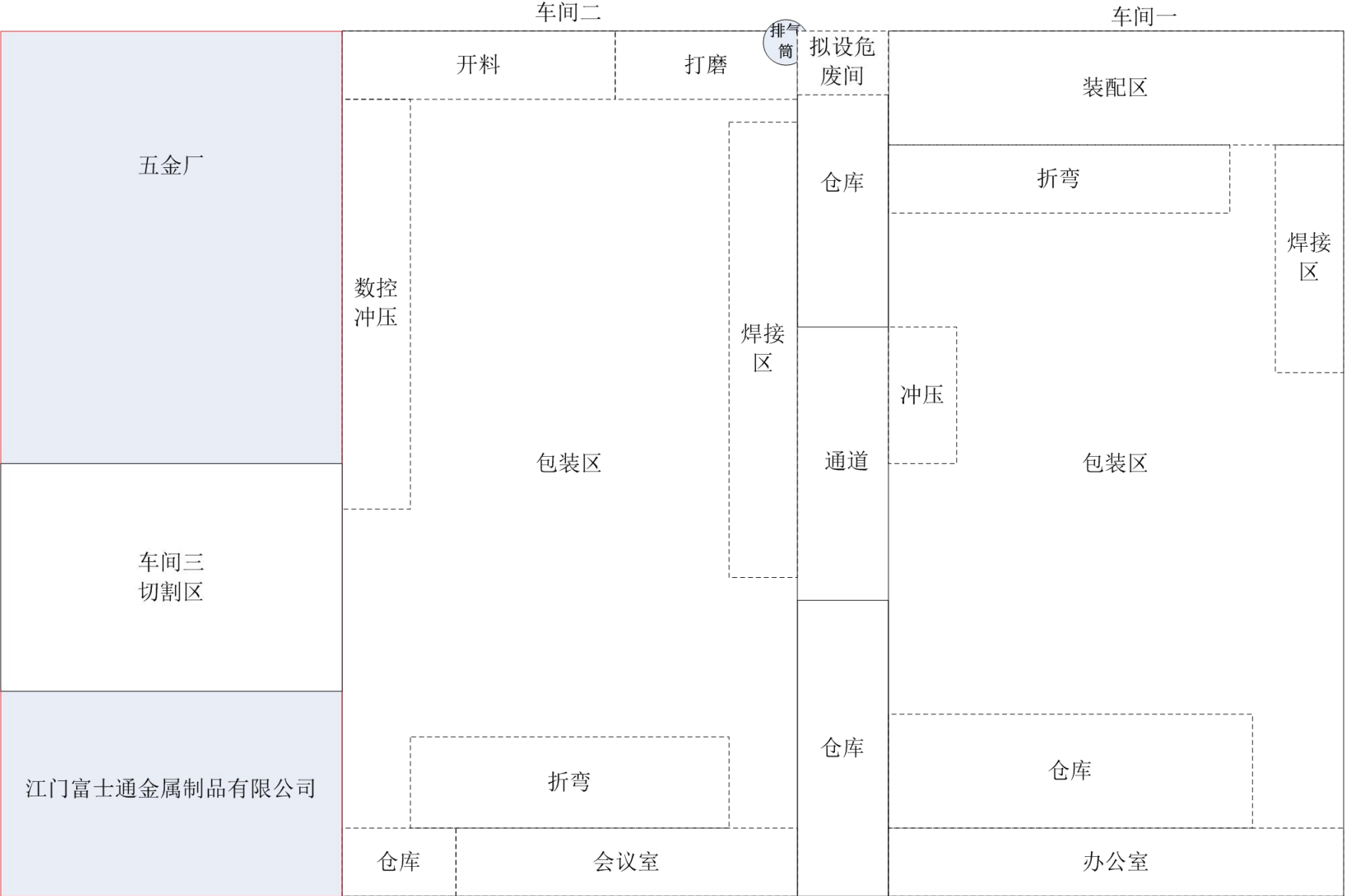
附图 4 厂房平面布置图
