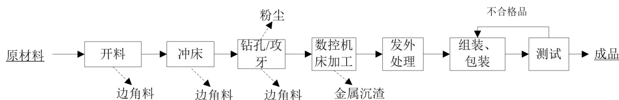
图 6-1 项目生产工艺流程图
