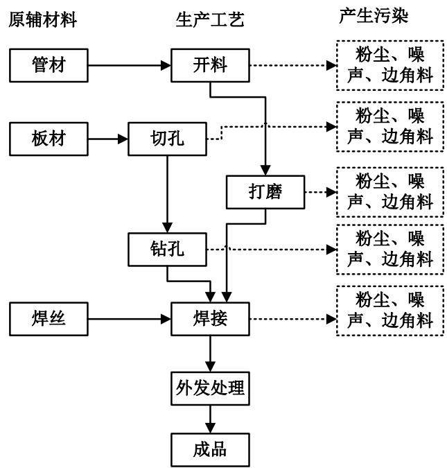
图 2-1 项目工艺流程图
