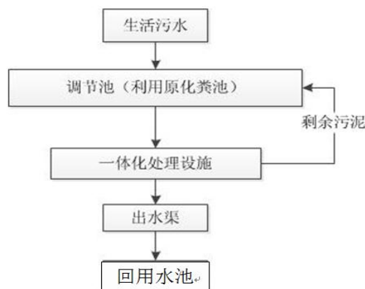
图 7-1 污水处理工艺流程图
