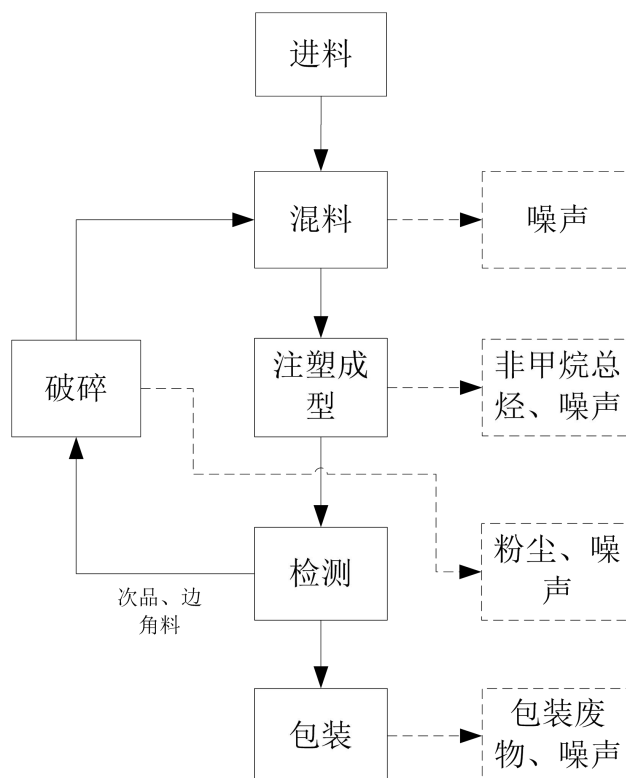
图 6-1 项目工艺流程图
