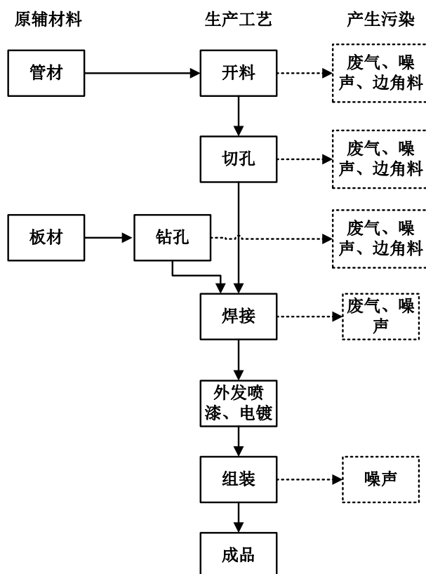
图 6-1 项目路灯生产工艺流程图
