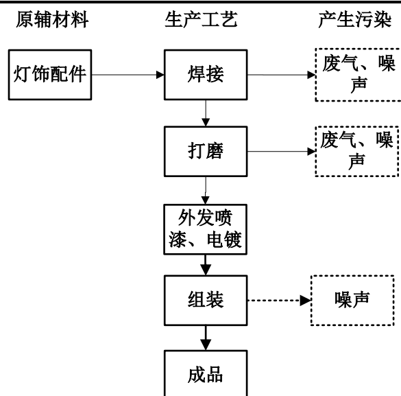
图2-2 项目灯饰生产工艺流程图
