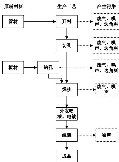
图 2-1 项目路灯生产工艺流程图
