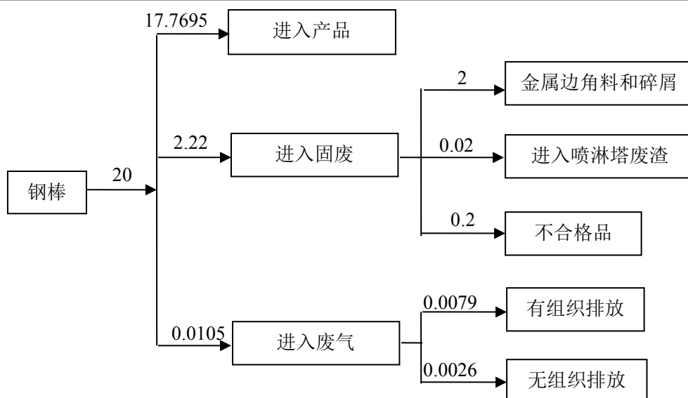
图 1-2 本项目物料平衡 (t/a)
