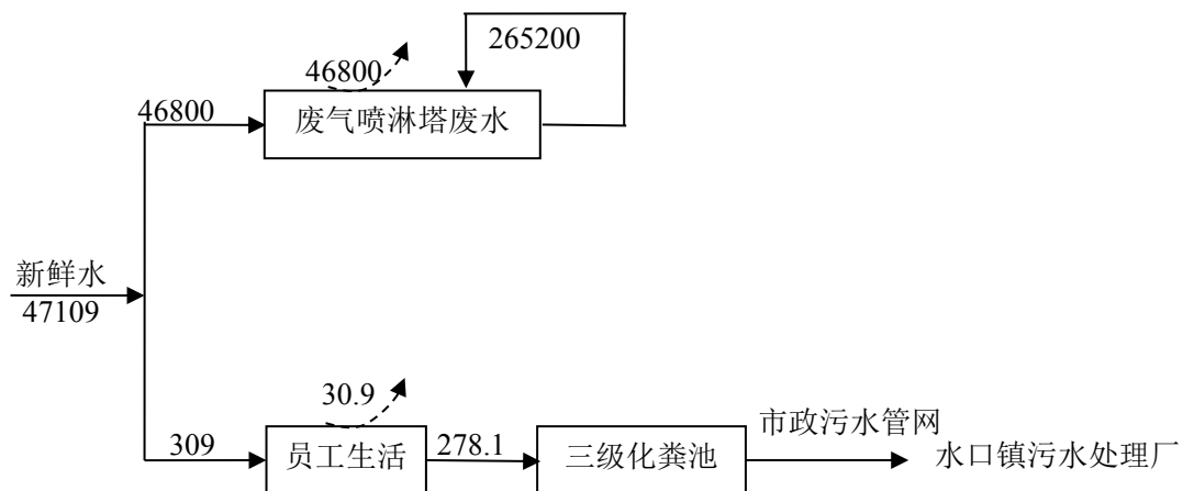
图 1-1 项目水平衡图（m³/a）
