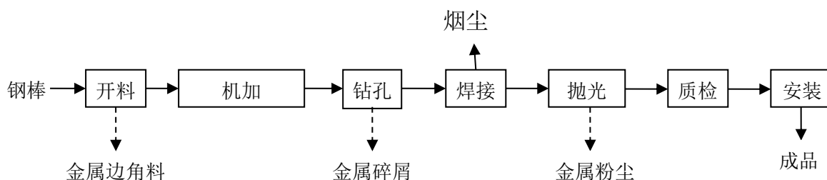
图 5-1 项目生产工艺流程图
