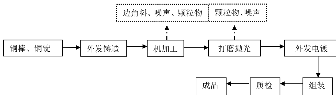
图 5-1 生产工艺流程图
